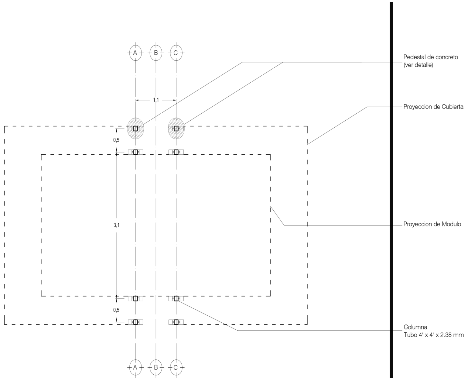
PLANTA DE DISTRIBUCION DE PEDESTALES
