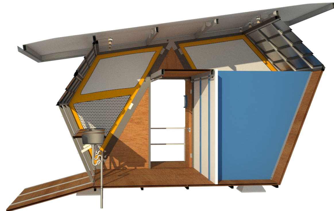
▼ Imagen N° 102. Corte espacial del MAD-Sanitario con tres duchas y tres lavamanos o pilas. Autoría propia.
