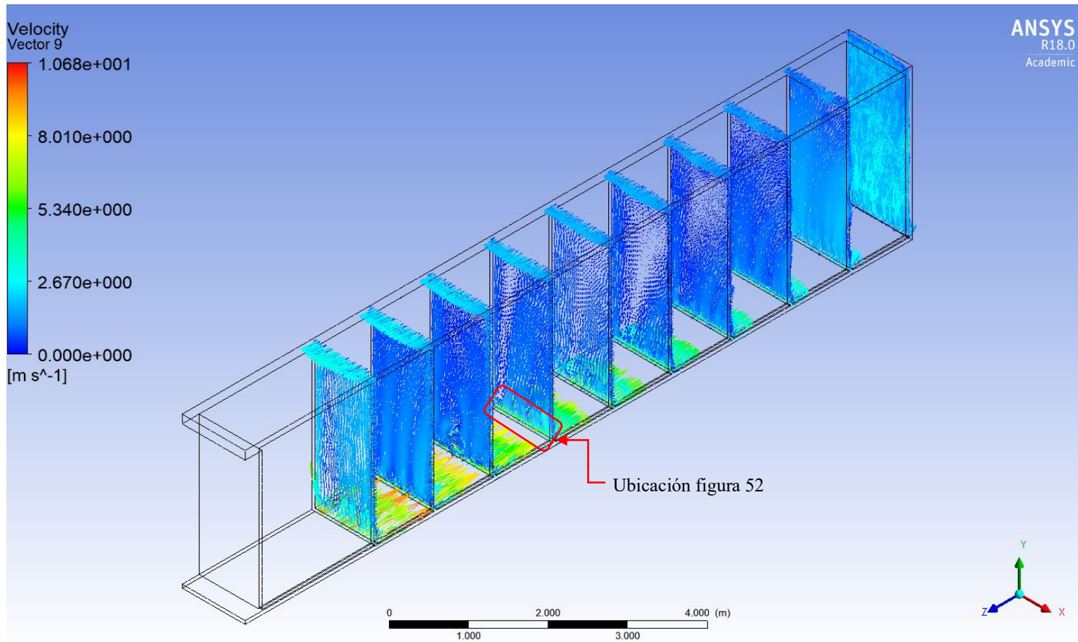
Figura 51. Recreación de vectores del flujo de aire frío en el espaciado entre columnas de cajas.
