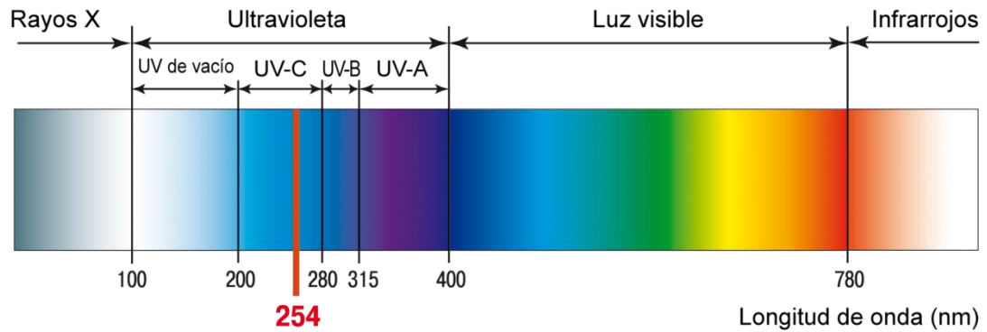
Figura 2-4 Espectro electromagnético [19].
