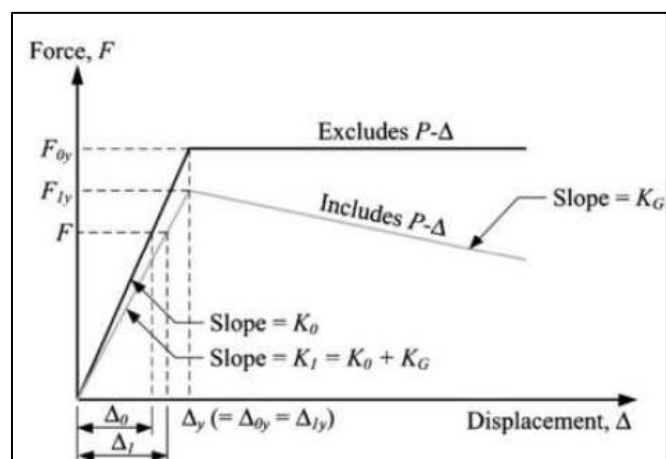
Figura 2.6. Respuesta idealizada de una estructura de un nivel con y sin el efecto P-Delta.
