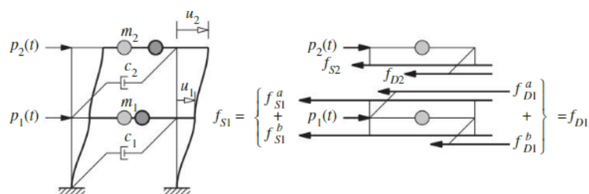
Figura 2.1. Marco de corte de dos niveles y las fuerzas que actúan sobre las dos masas.
