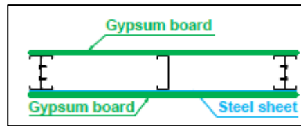
Figura 5.3. Sección de sistema de gypsum para pared liviana.
