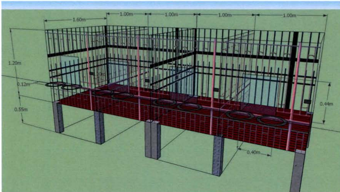
Figura 11. Diseño de ternerera elaborado para la finca Asociación Roblealto. (2013)
