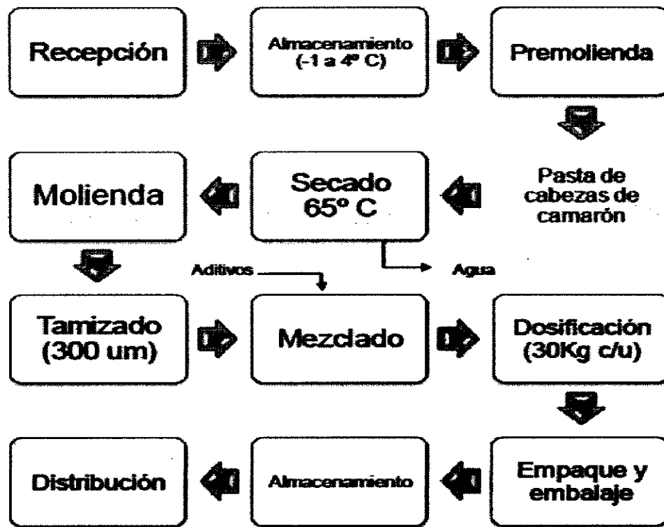
Figura 1. Diagrama de flujo para la elaboración de una harina de camarón para consumo animal según Chavéz et al. 2010.
